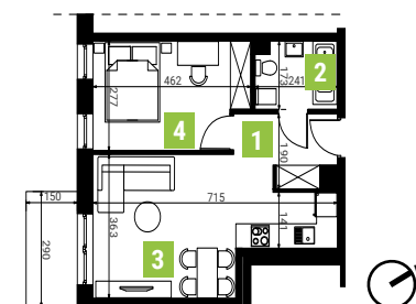
Rzut mieszkania
