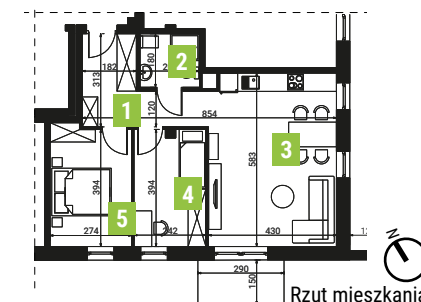
Rzut mieszkania
